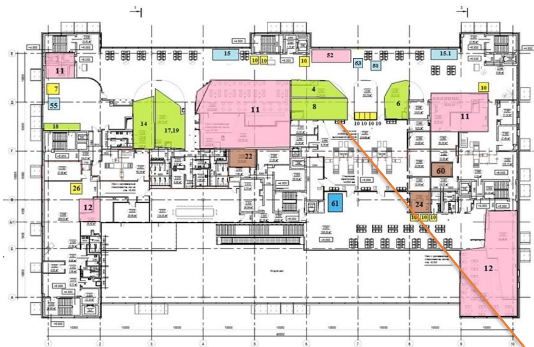
План 2-го этажа (на отм. +6.000), М 1:200
